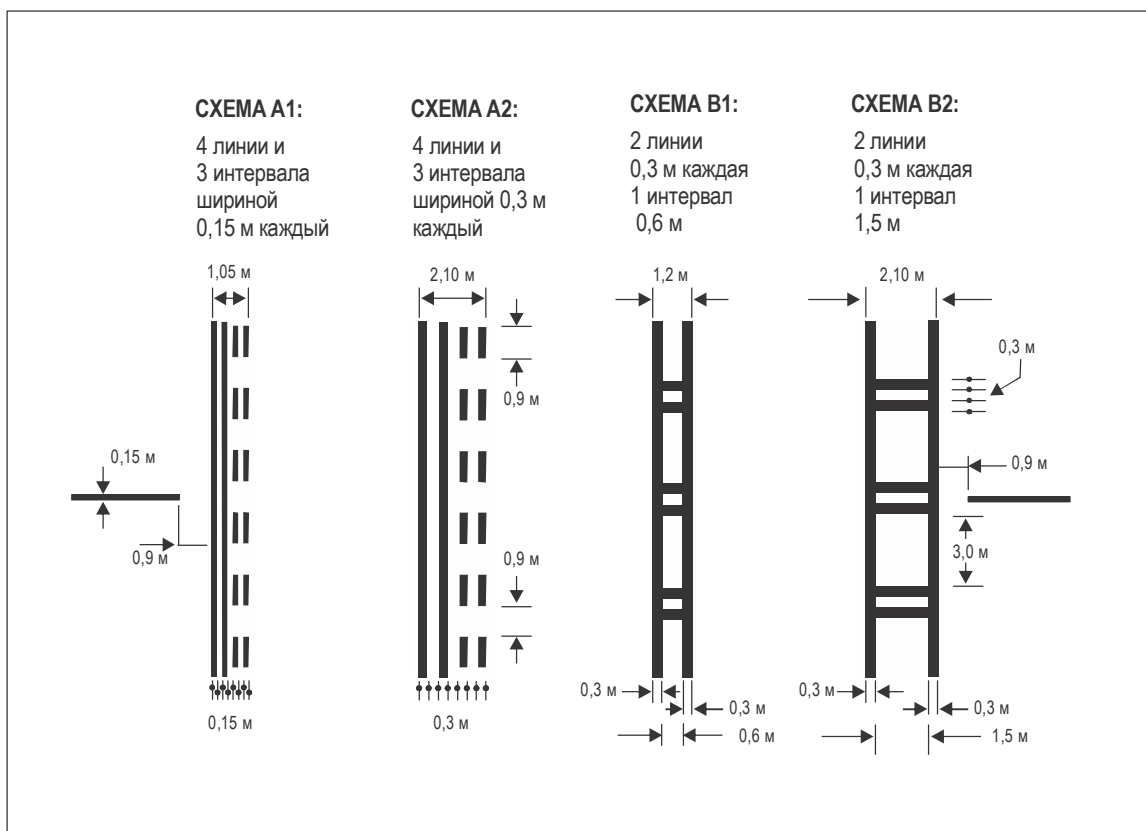
Рис. 5-8. Маркировка места ожидания у ВПП Примечание. После 2026 года схемы А1 и В1 применяться не будут.
