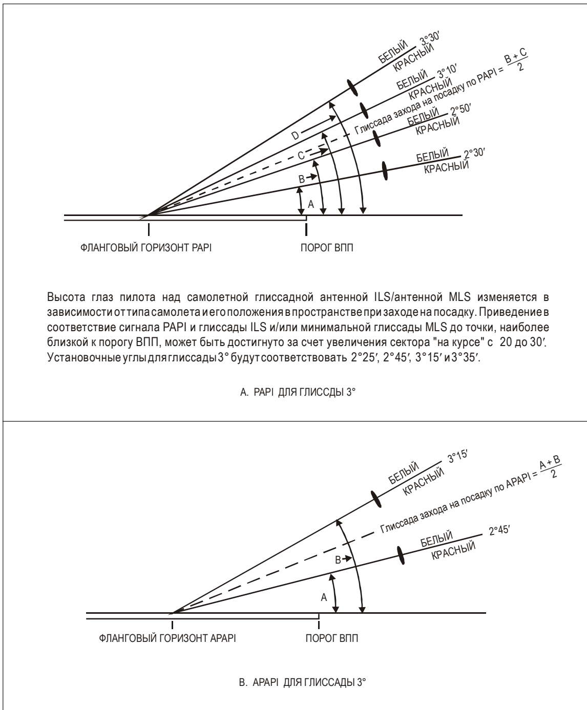
Рис. 5-20. Световые лучи и установка углов возвышения PAR1 и ARAP1
