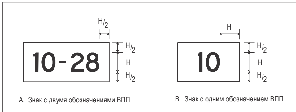
Рис. А4-4. Размеры знака
