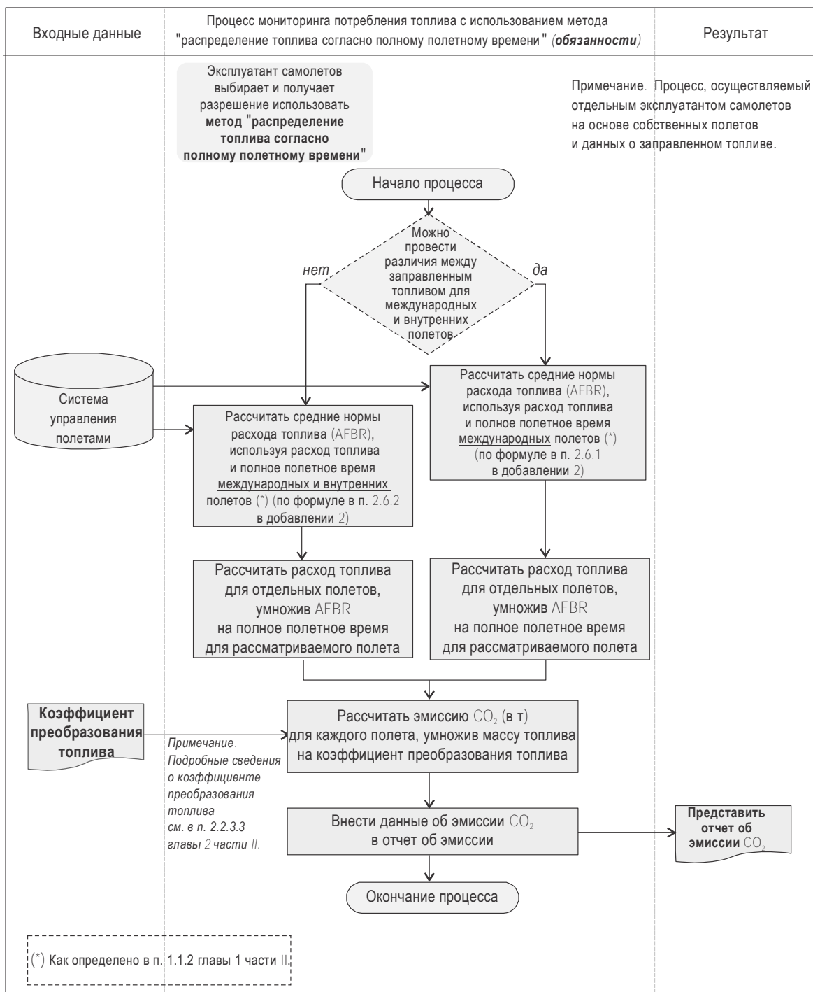
Рис. С-8. Мониторинг потребления топлива за полет с использованием метода "распределение топлива согласно полному полетному времени"
