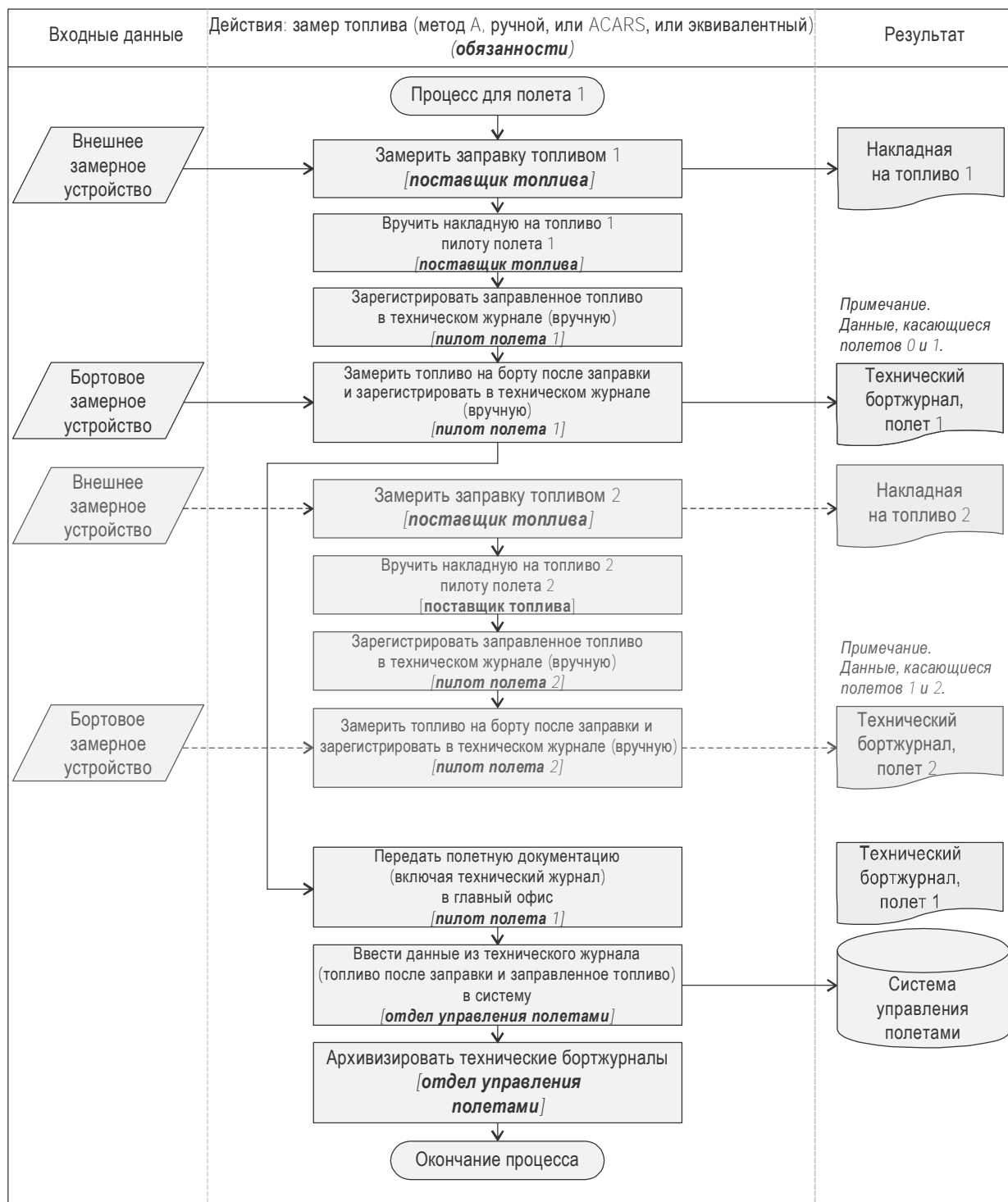
Рис. С-2. Сбор требуемых данных для применения метода А с заправленным топливом от поставщика топлива
