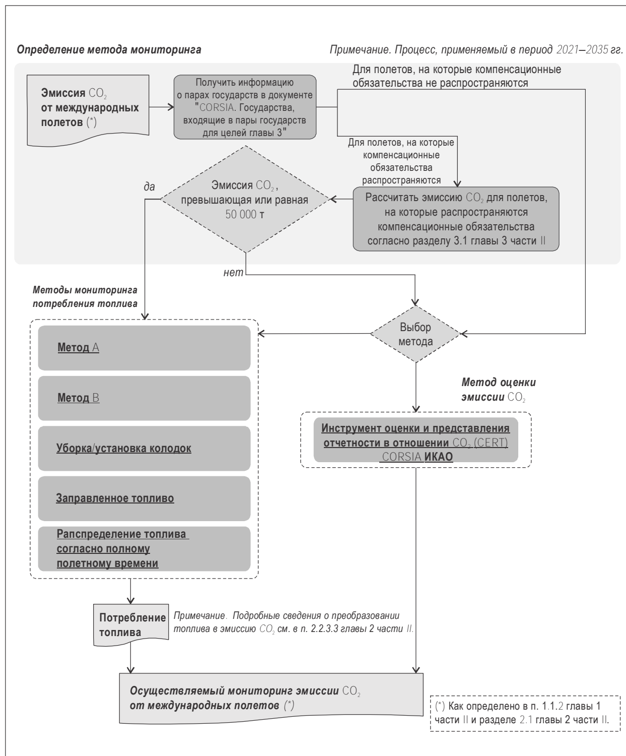
Рис. В-3. Определение применимых методов мониторинга потребления топлива в течение периодов соблюдения условий (2021–2035 гг.)
