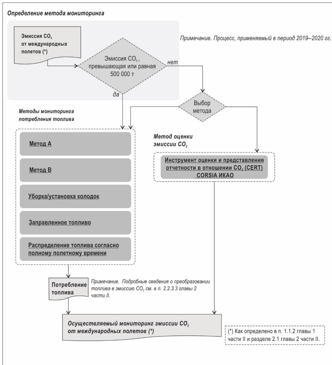
Рис. В-2. Определение применимых методов мониторинга потребления топлива в период 2019–2020 гг.
