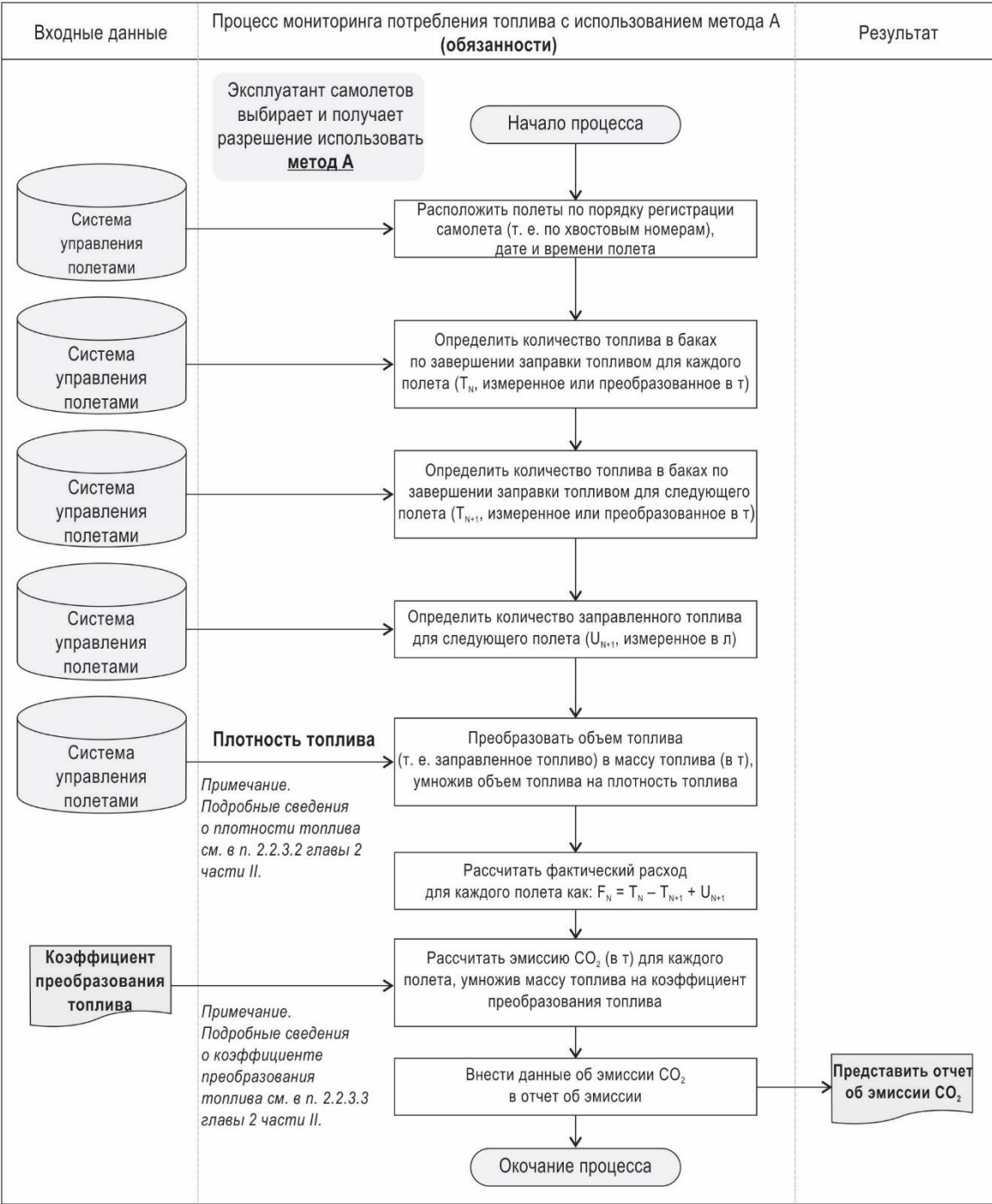
Рис. С-1. Мониторинг потребления топлива за полет с использованием метода А
